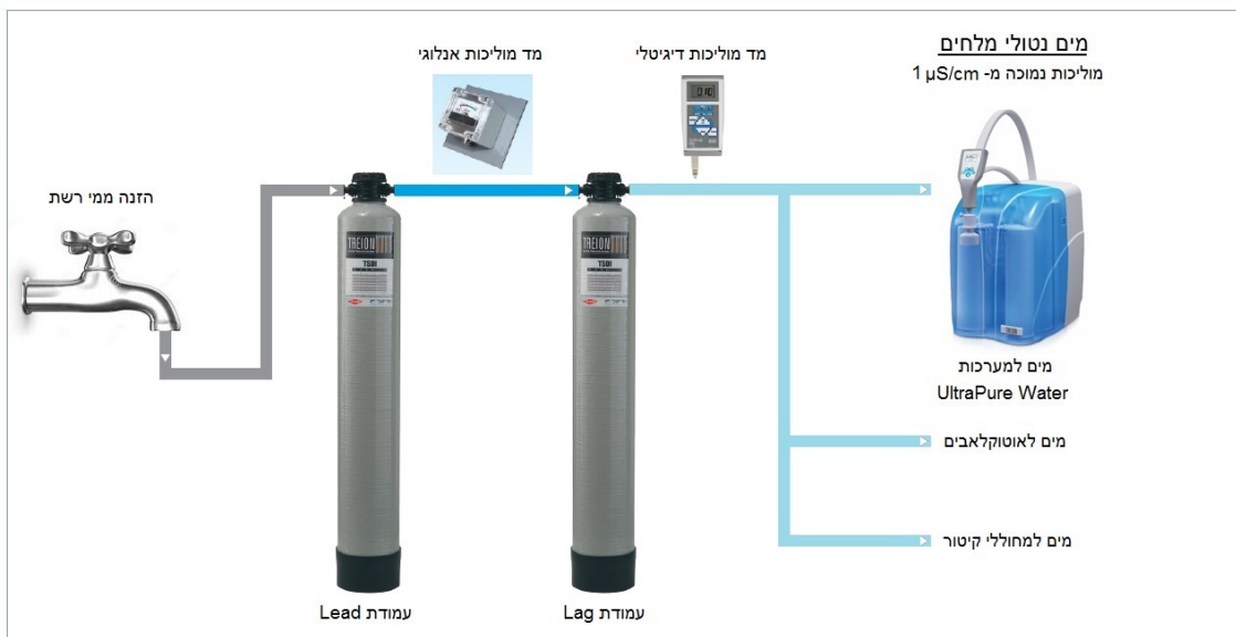
דוגמה להתקנת Lead-Lag
